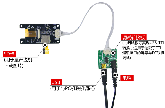
图 1-3 调试工具图
